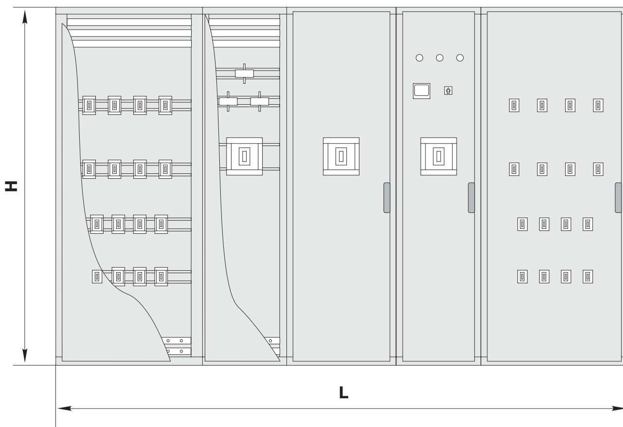
Рис. 20.2 Габаритные размеры главного распределительного щита серии ГРЩ
