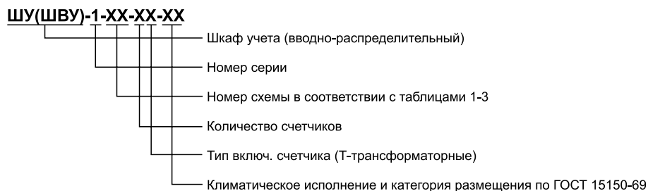
Рис. 4.1 Структура условного обозначения шкафов серии ШВУ-1
