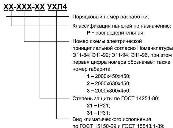
Рис. 2.2 Структура условного обозначения распределительных панелей устройств серии ВРУ85хх
