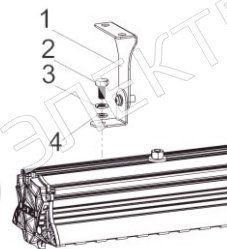
Рисунок 4 Монтаж крепления
