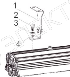
Рисунок 4 Монтаж крепления
