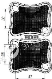
Рисунок 1б Светильник «L-one». Сдвоенный вариант
