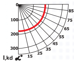
Кривая силы света (М) НББ64-60-066
